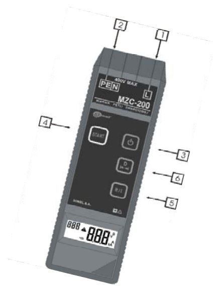
Рис.1. Расположение гнёзд и клавиш в измерителях семейства MZC-200 (лицевая панель)
