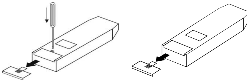
Рис.4. Вскрытие отсека элементов питания в приборах семейства MZC-200
