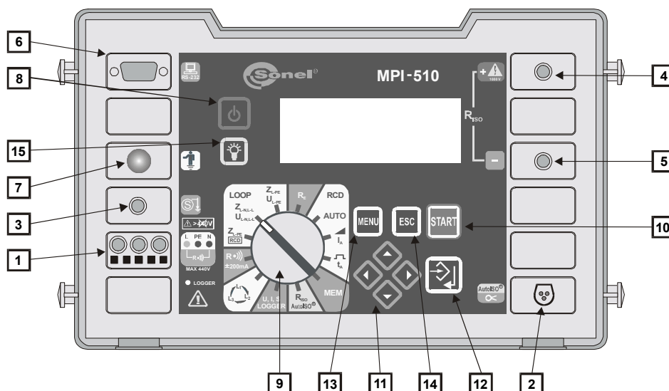
Рис.1. Размещение гнезд и клавиш измерителя MPI-510 (лицевая панель).
