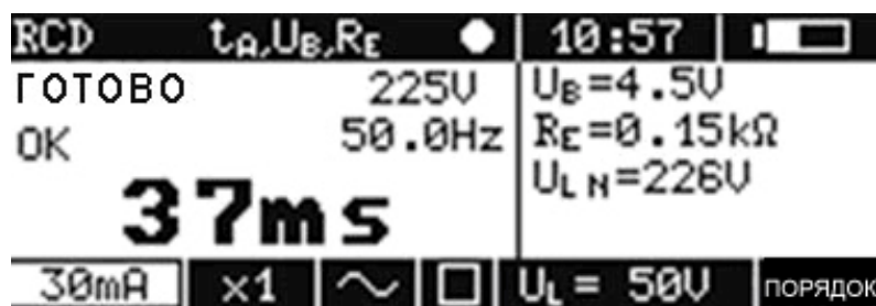
Рис.20. Вид экрана при измерении времени отключения УЗО
