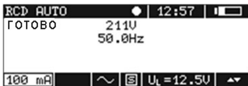
Рис.21. Организация экрана при автоматическом измерении УЗО
