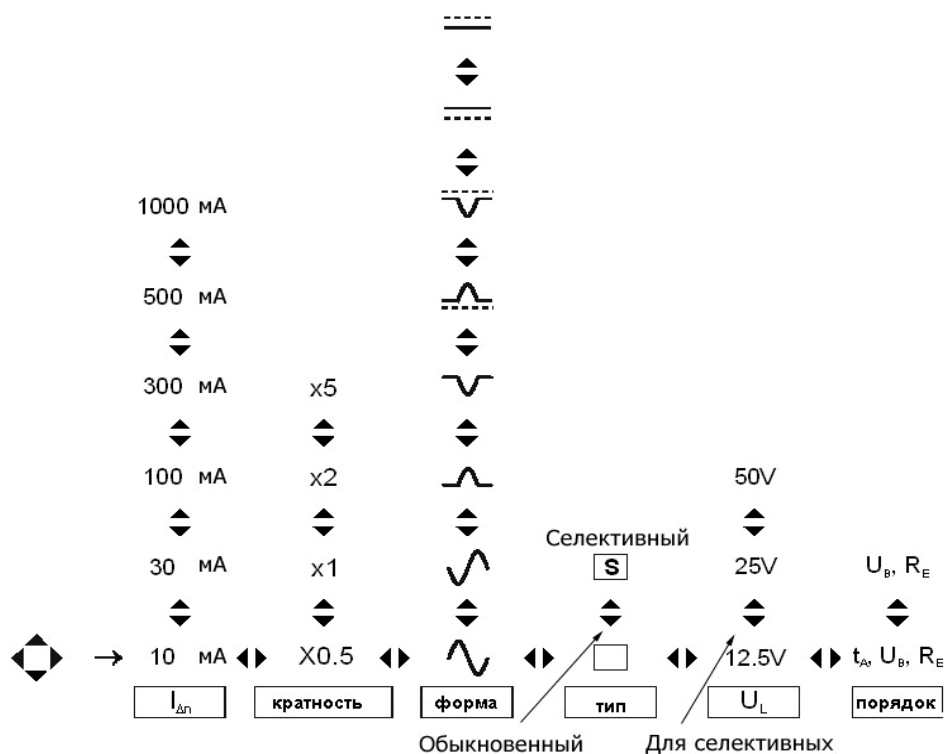
Рис.19. Отображение параметров измерения t_d
