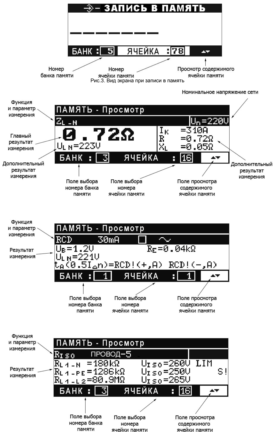
Рис.4. Вид экрана при просмотре памяти : а) результаты измерений сопротивления петли короткого замыкания (похожий вид имеет экран с результатами измерений сопротивления изоляции, сопротивления заземления и сопротивления, измеряемого током с низким напряжением \pm 200 mA), б) результаты измерений параметров УЗО (знак RCD! означает, что измерения проводятся без срабатывания УЗО, символы +/- - фазу или поляризацию положительную/отрицательную, буква A означает замер, выполненный в режиме (AUTO)), в) результаты измерений сопротивления изоляции многожильных проводов.
