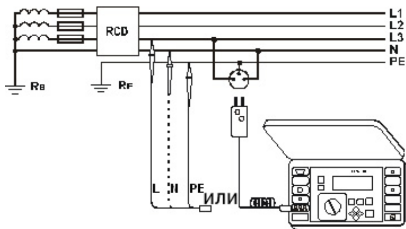
Рис.16. Измерение в цепи, оснащенной УЗО, при помощи зондов с острием или при помощи зонда в виде вилки (нулевой провод нужен только для тока ( I_{\Delta n} ) постоянного и пульсирующего, его отсутствие сигнализируется сообщением на дисплее.
