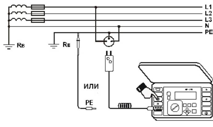
Рис. 6. Проверка правильности подключения защитного провода
