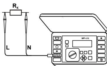
Рис.35. Измерение сопротивления низким напряжением
