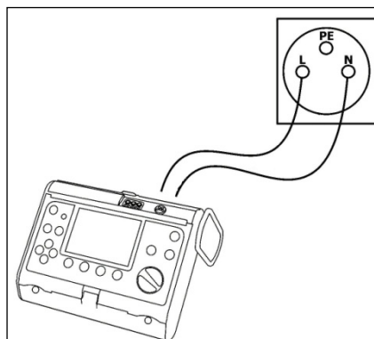
Рис.5. Подключение измерителя.
