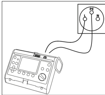
Рис.19. Подключение прибора.
