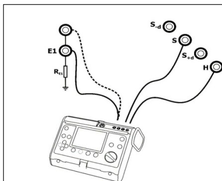
Рис.8 Подключение измерителя.
